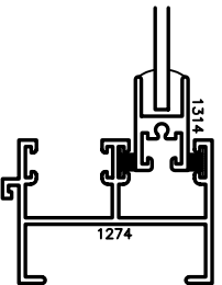
② JAMB
