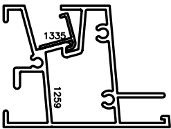
OPTIONAL SILL
