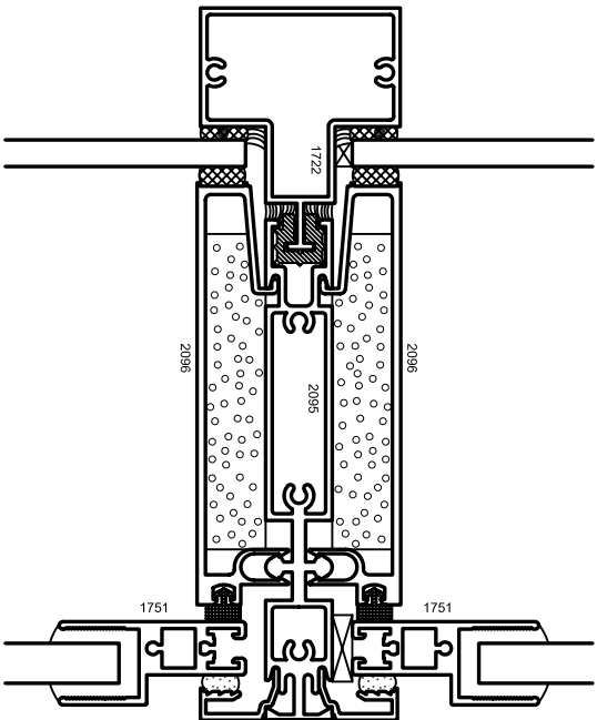
OPTIONAL T-BAR
