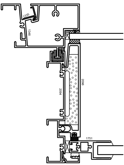
OPTIONAL SILL
