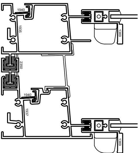
OPTIONAL SASH SILL
