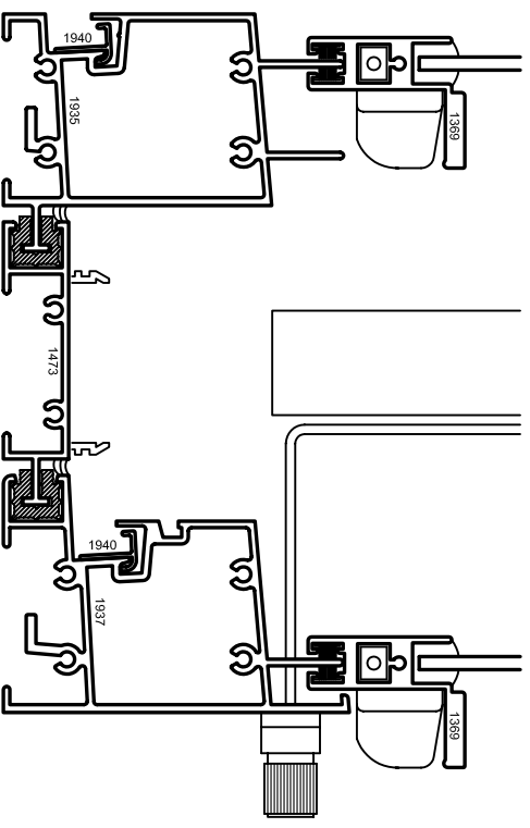
OPTIONAL SASH SILL
