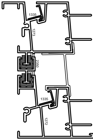
OPTIONAL SILL
