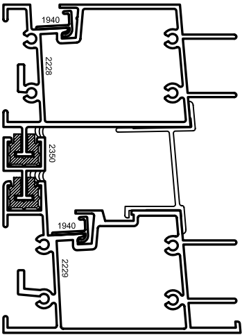
OPTIONAL SILL
